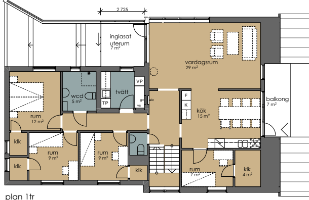
plan 1tr
